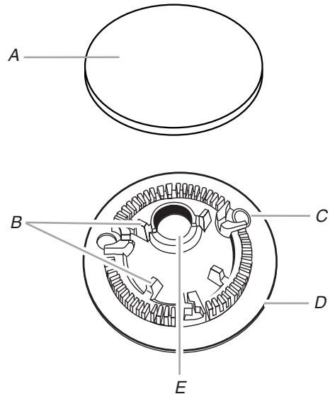
A. Tapa del quemador B. Espigas de alineación C. Encendedor D. Quemador E. Abertura del tubo de gas
